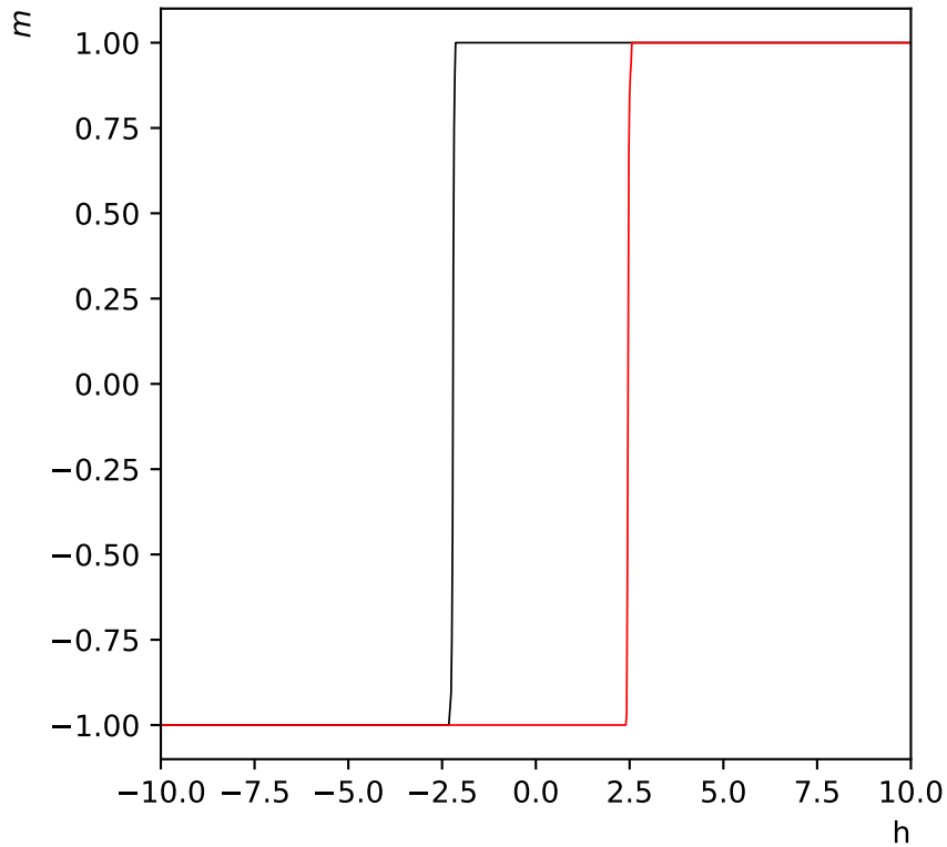
Hystérésis de l'aimantation réseau de taille L=8 - h=10 à T=0.5
