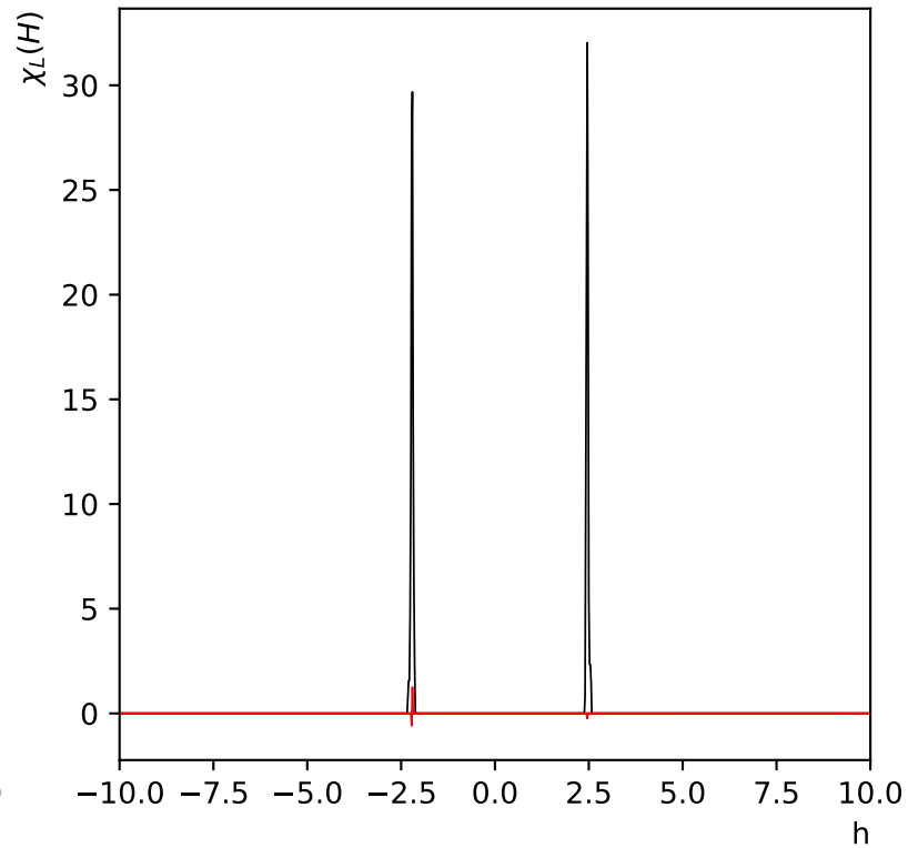
\chi_L(H) réseau de taille L=8 à T=0.5
